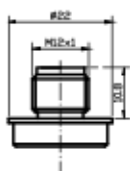
Разъем M12x1 (S763) (IP67)
