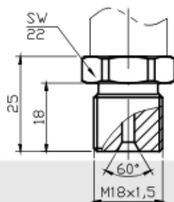
M18x1,5
