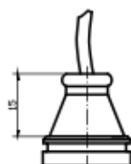
Кабель (IP67/IP69K)
