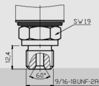
9/16-18 UNF-2A / IK 60°
