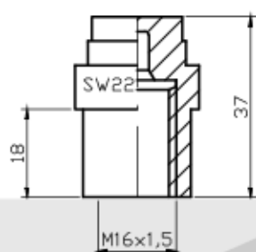
M16x1,5 Внутр.
