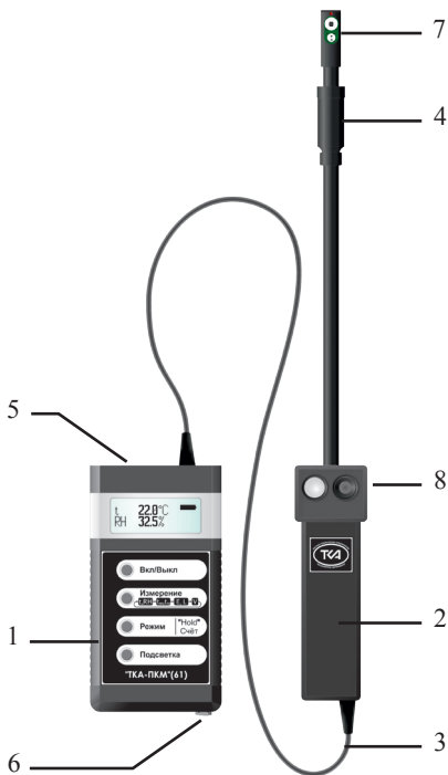
Рис.1. Внешний вид прибора “ТКА-ПКМ”(61)
