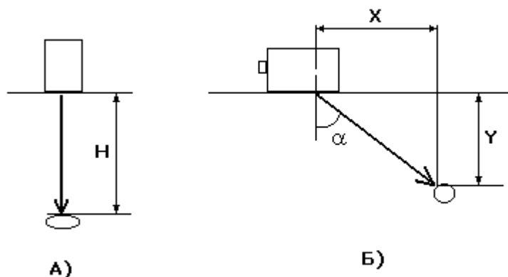
Рис. 4.12.1. Схемы прозвучивания отражателей и обозначение координат дефекта. 10) прямым преобразователем. Б) наклонным преобразователем.
