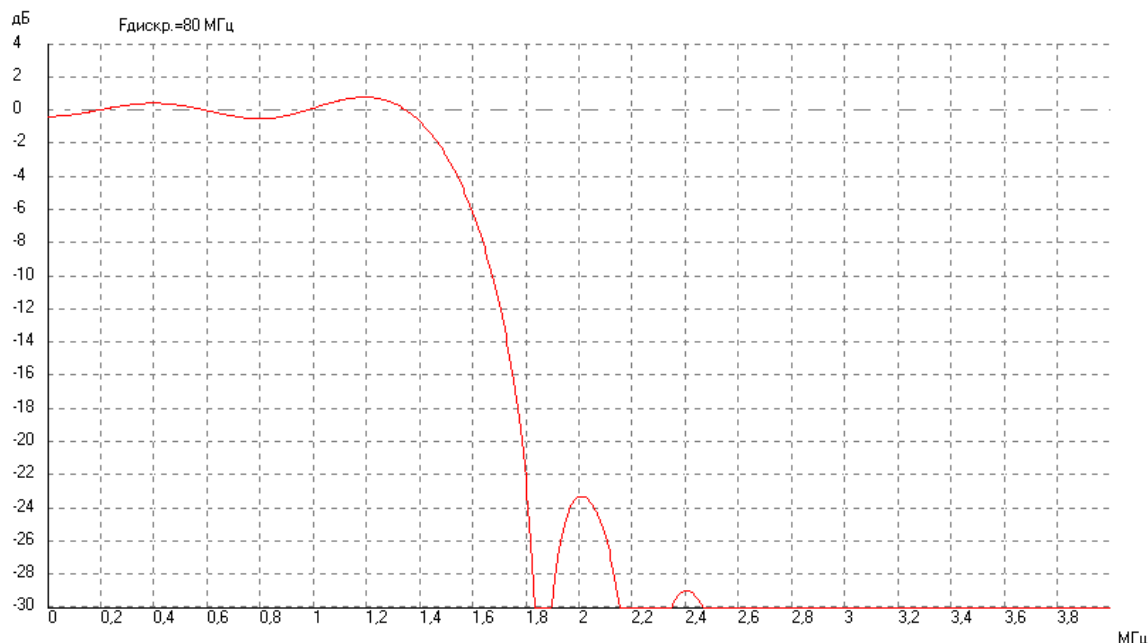
Рис. 4.4.4. Амплитудно-частотная характеристика цифрового фильтра нижних частот с частотой среза 1,5 МГц.
