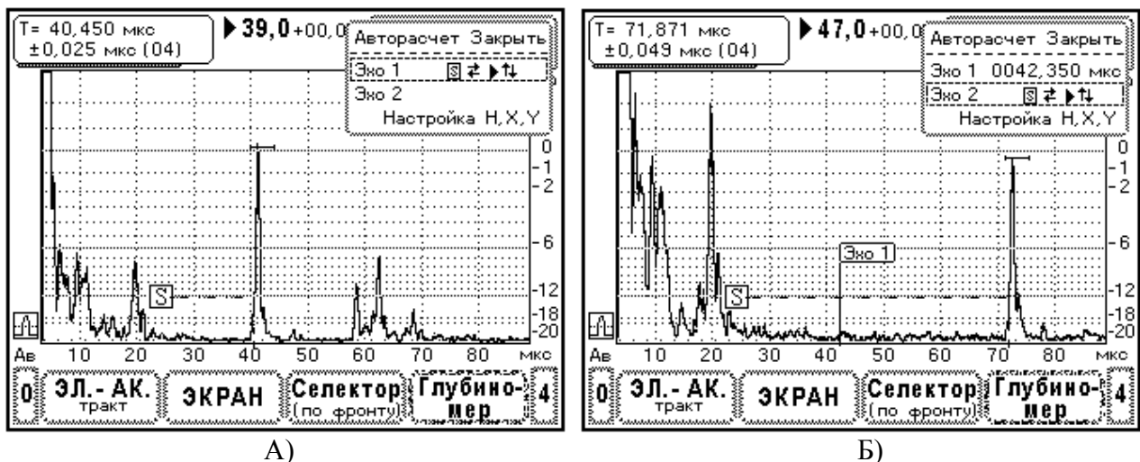
Рис. 9.4.5.2. Измерение задержки эхосигналов в СОП.
