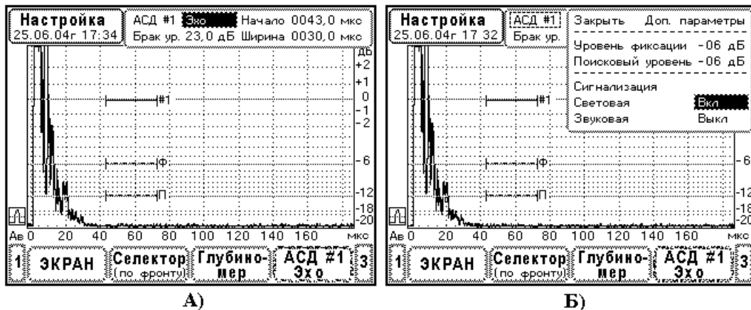
Рис. 9.4.10.1. Меню АСД#1.
