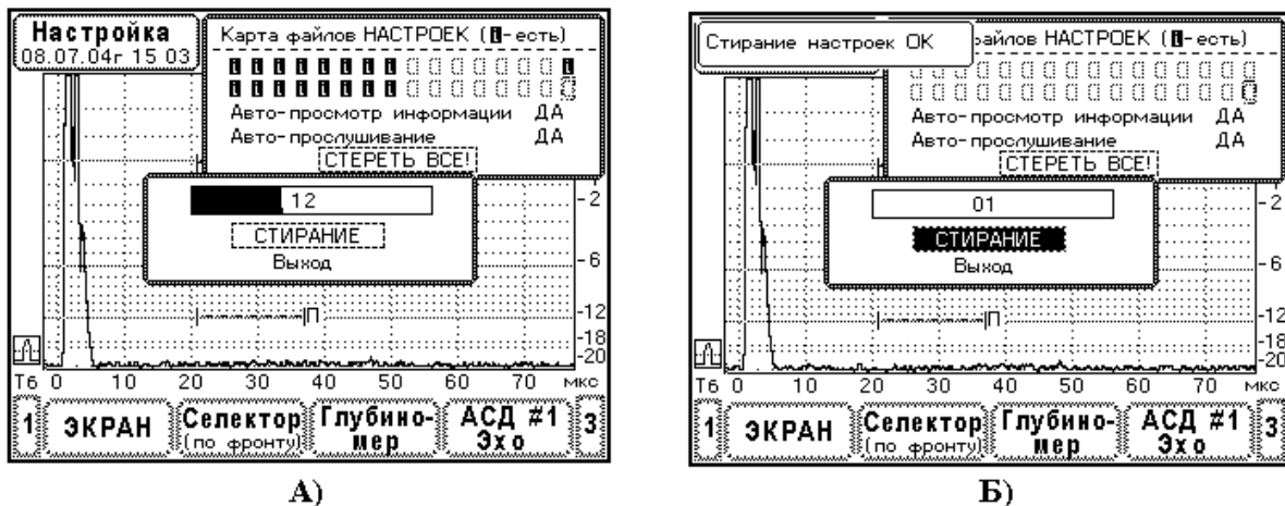
Рис. 9.4.17.5. Стирание настроек.
