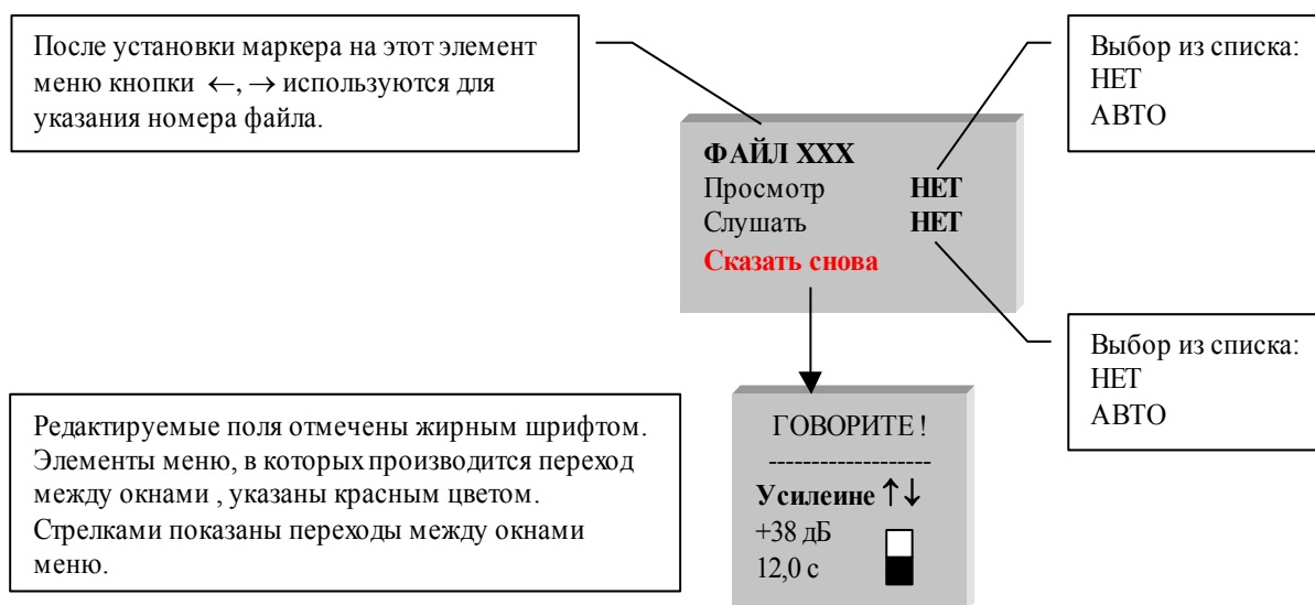
Рис. 8.1.1. Структура управляющего меню «Файл XXX».
