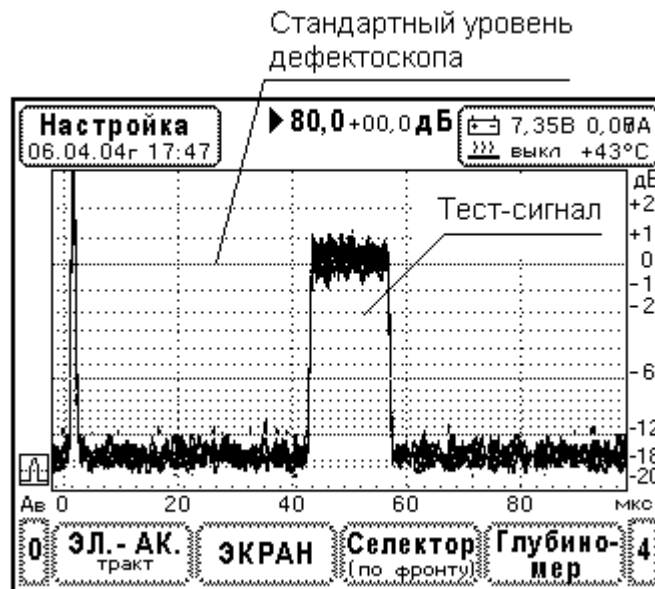
Рис.10.6.4.3. Вид тест-сигнала при измерении максимальной чувствительности приемника дефектоскопа.
