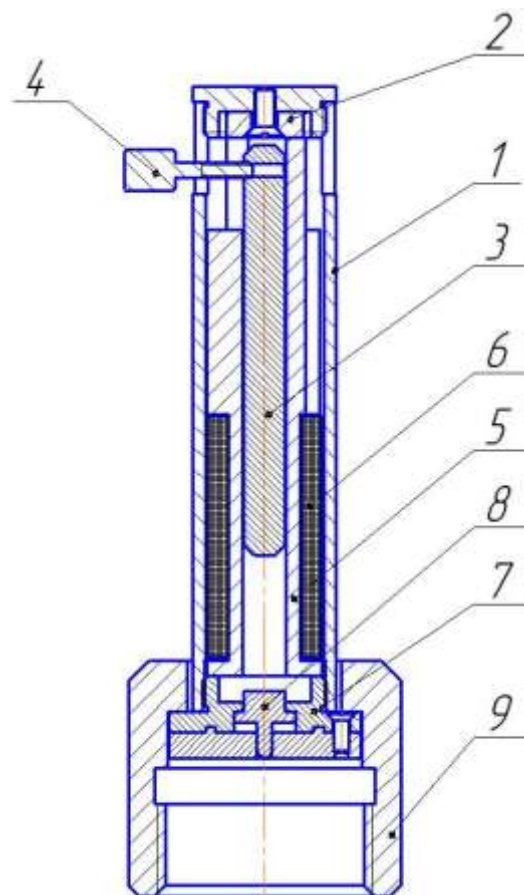
Рис.3. Общий вид.
