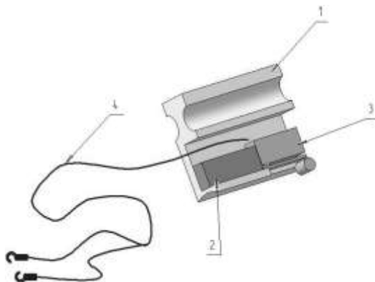
Рис.6. Общий вид.
