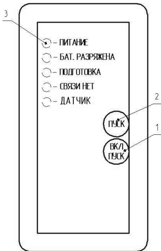
Рис.4. Пульт управления ПУ.
