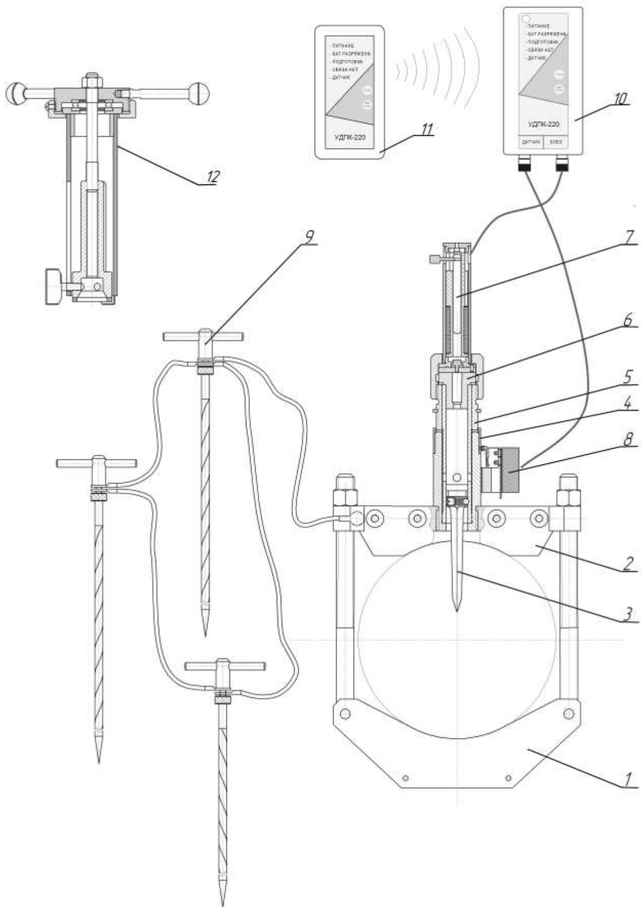
Рис.1 Общий вид УПКП 130, 200.
