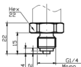
G 1/4" B
