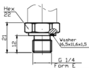
G 1/4" A; Форма E
