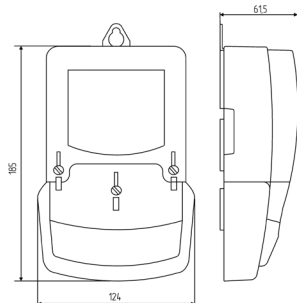
Рисунок А.3 – Габаритные и установочные размеры счетчика СЕ 200 S10
