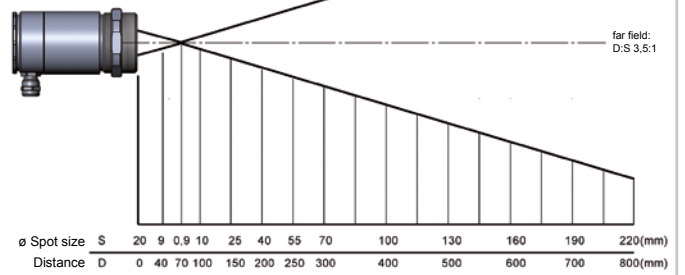
CF1 optics 75:1
