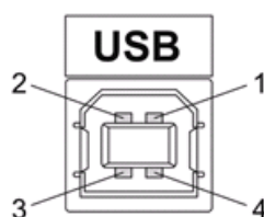
Рисунок 3.10 Разъем USB (розетка «В»)
