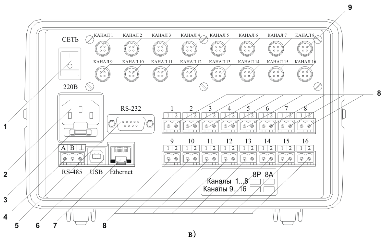
Рисунок 3.7 Вид задних панелей приборов ИВТМ-7 /4(8,16)-Т-ХР-УА (7): а – четырехканального исполнения б- восьмиканального исполнения в - шестнадцатиканального исполнения
