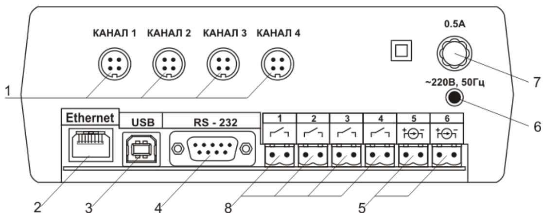
Рисунок 3.4 Вид задних панелей приборов ИВТМ-7 /X-T-4P-2A-E (3):
