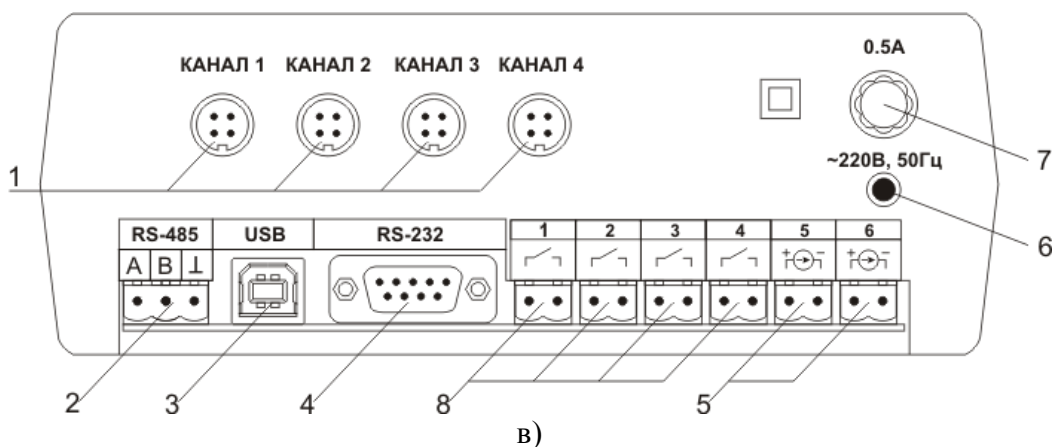
Рисунок 3.3 Вид задних панелей приборов ИВТМ-7 /X-T-4P-2А (3):
