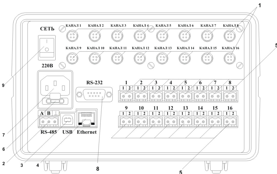
Рисунок 3.6 Вид задней панели приборов ИВГ-1 /8-Т-УР-ZA (7):
