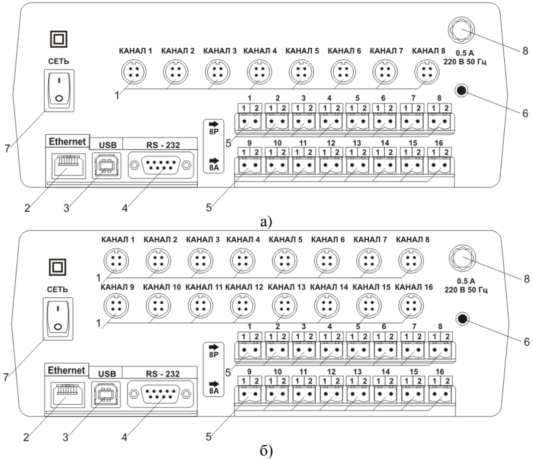
Рисунок 3.4 Вид задних панелей приборов ИВГ-1 /4(8)-Т-8Р-8А-Е : а - четырехканального исполнения б - восьмиканального исполнения
