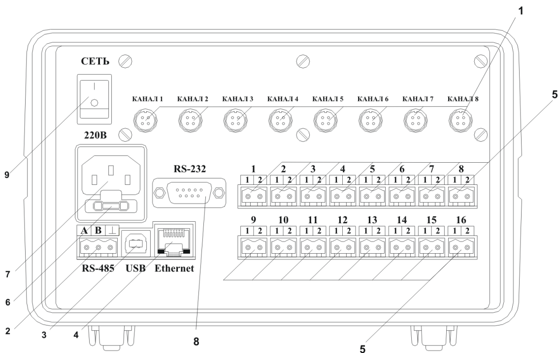
Рисунок 3.5 Вид задней панели приборов ИВГ-1 /4-Т-УР-ZA:
