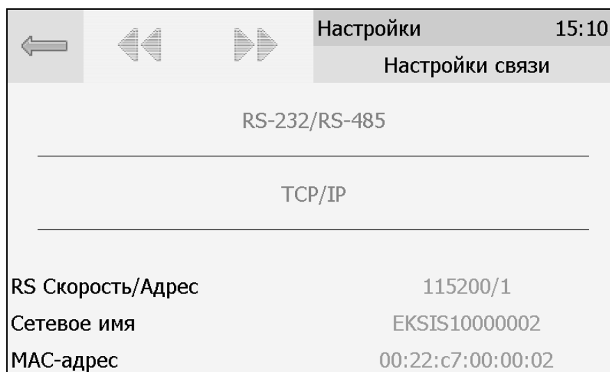
Рисунок 6.27 Экран настроек связи (ИБГ-1 /X-T-XP-УА)
