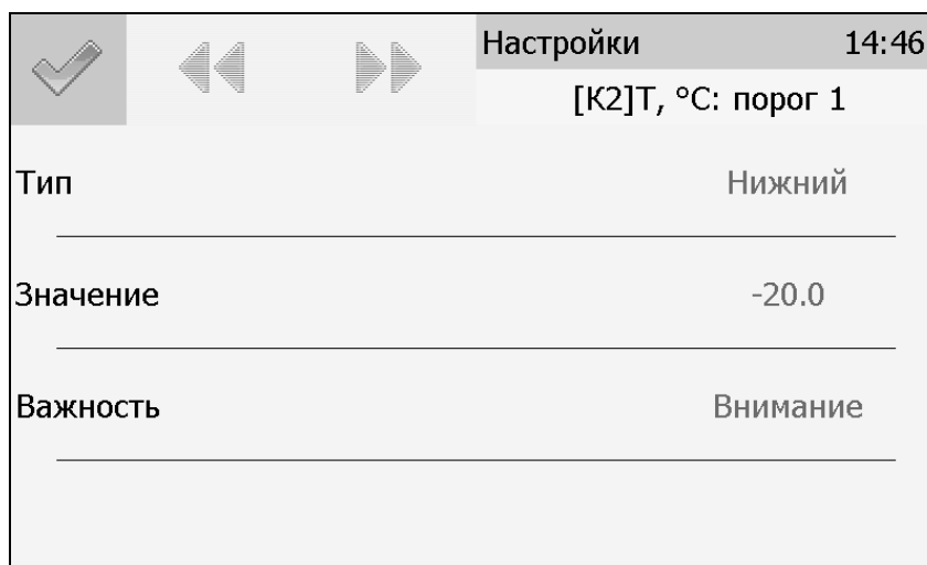
Рисунок 6.5 Экран настройки первого порога для температуры
