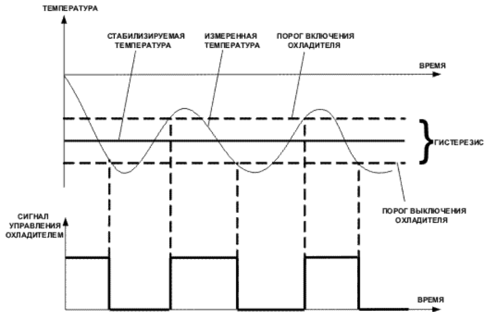
Рисунок 3.17 Диаграмма работа стабилизаторов температуры с гистерезисом в случае управления охладителем
