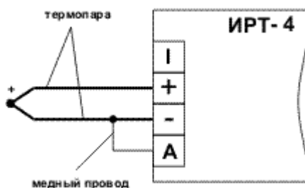
Рисунок 3.13 Прямое подключение термопары
