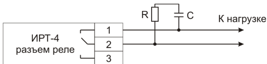
Рисунок 3.21 Подключение выходных устройств с реле
