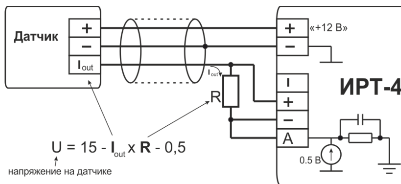
в) трехпроводная схема с использованием внутреннего источника питания «12В»
