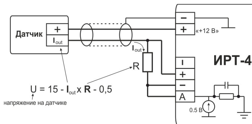
а) двухпроводная схема с использованием внутреннего источника питания «12В»
