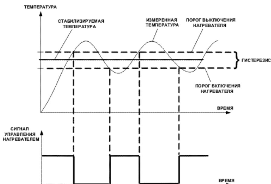
Рисунок 3.16 Диаграмма работа стабилизаторов температуры с гистерезисом в случае управления нагревателем
