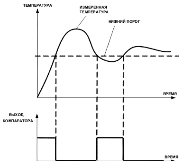
Рисунок 3.19 Диаграмма работа компаратора нижнего порога
