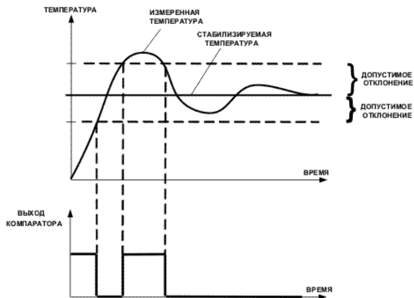
Рисунок 3.18 Диаграмма работа компаратора допустимого отклонения
