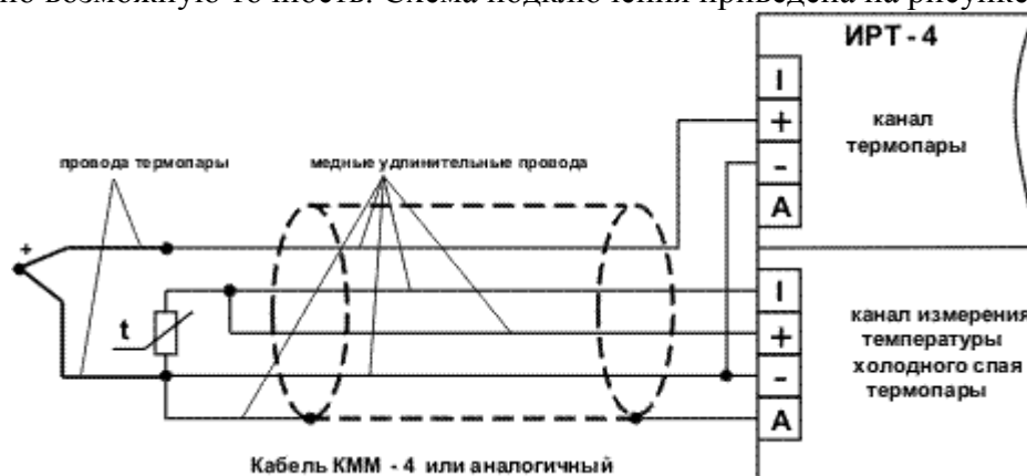
Рисунок 3.12 Подключение термопары с помощью удлинительных проводов
