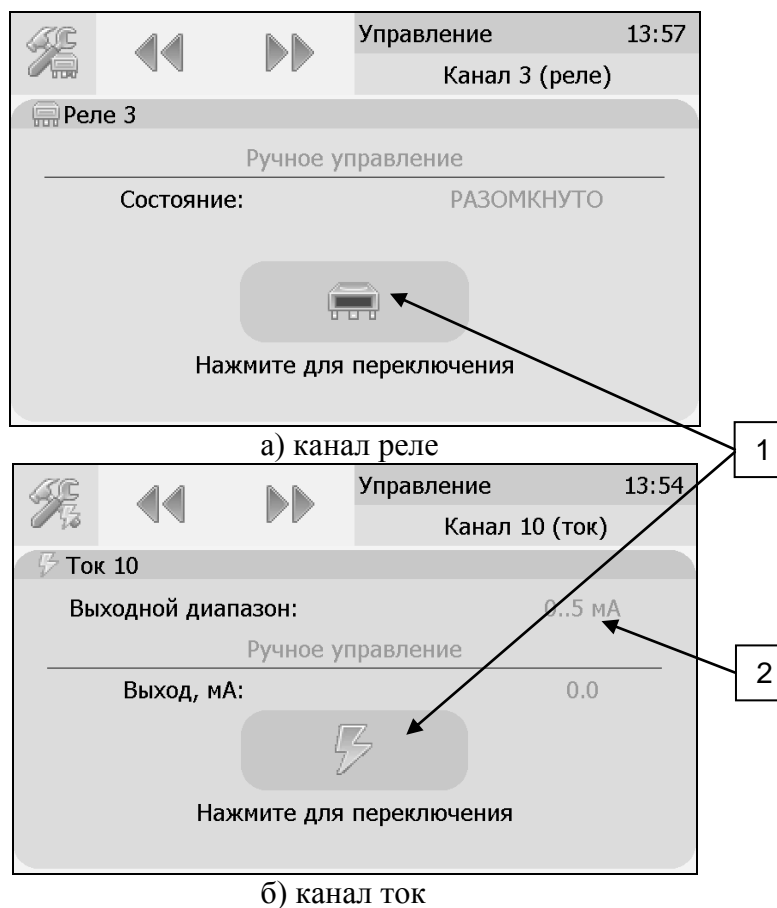
Рисунок 6.10 Виды экрана первого и пятого канала управления
