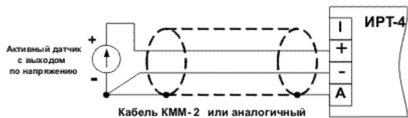
Рисунок 3.14 Подключение активного датчика с выходом по напряжению
