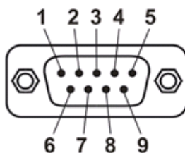
Рисунок 3.4 Разъем подключения к компьютеру по RS-232
