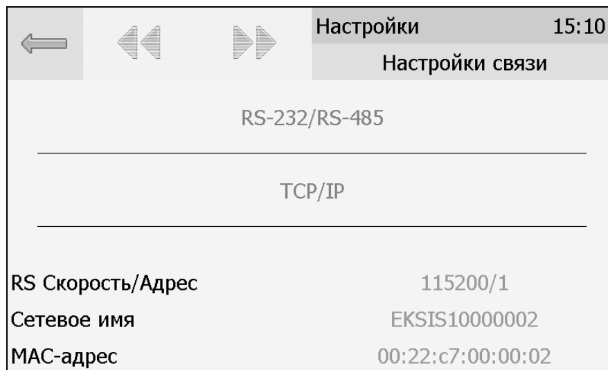
Рисунок 6.21 Экран настроек связи ИРТ-4/16-Т-ХР-УА
