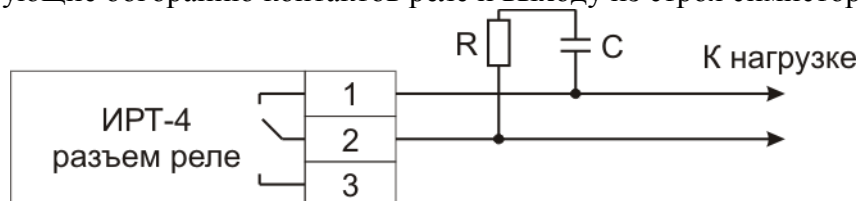
Рисунок 3.7 Подключение нагрузки к выходу управления
