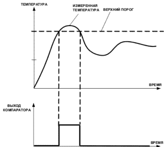
Рисунок 3.20 Диаграмма работа компаратора верхнего порога
