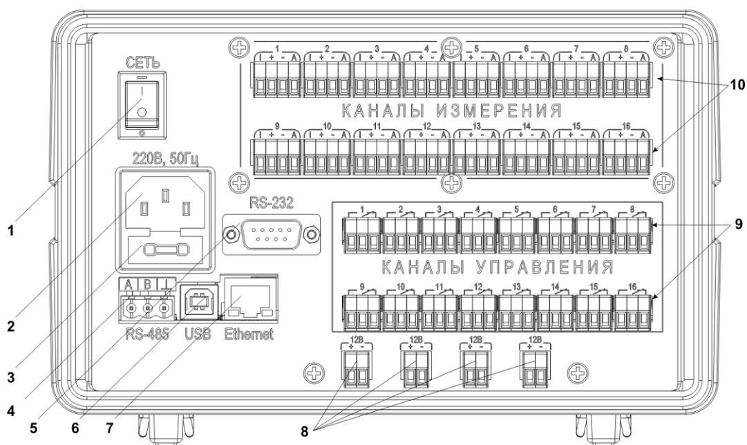
Рисунок 3.3 Вид задней панели измерителя-регулятора ИРТ-4/16-Т-ХР-УА:
