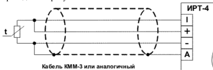
Рисунок 3.9 Четырехпроводная схема
