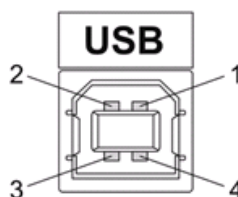
Рисунок 3.5 Разъем USB (розетка «B»)
