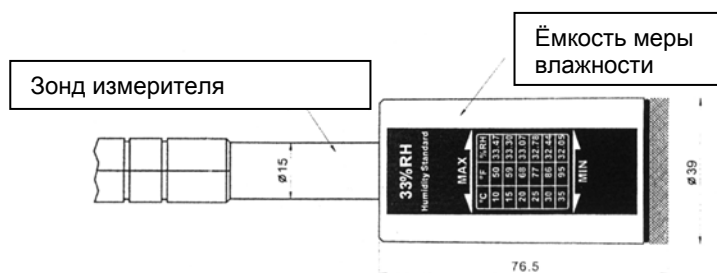
Рис.2 Схема соединения с измерителем Center
