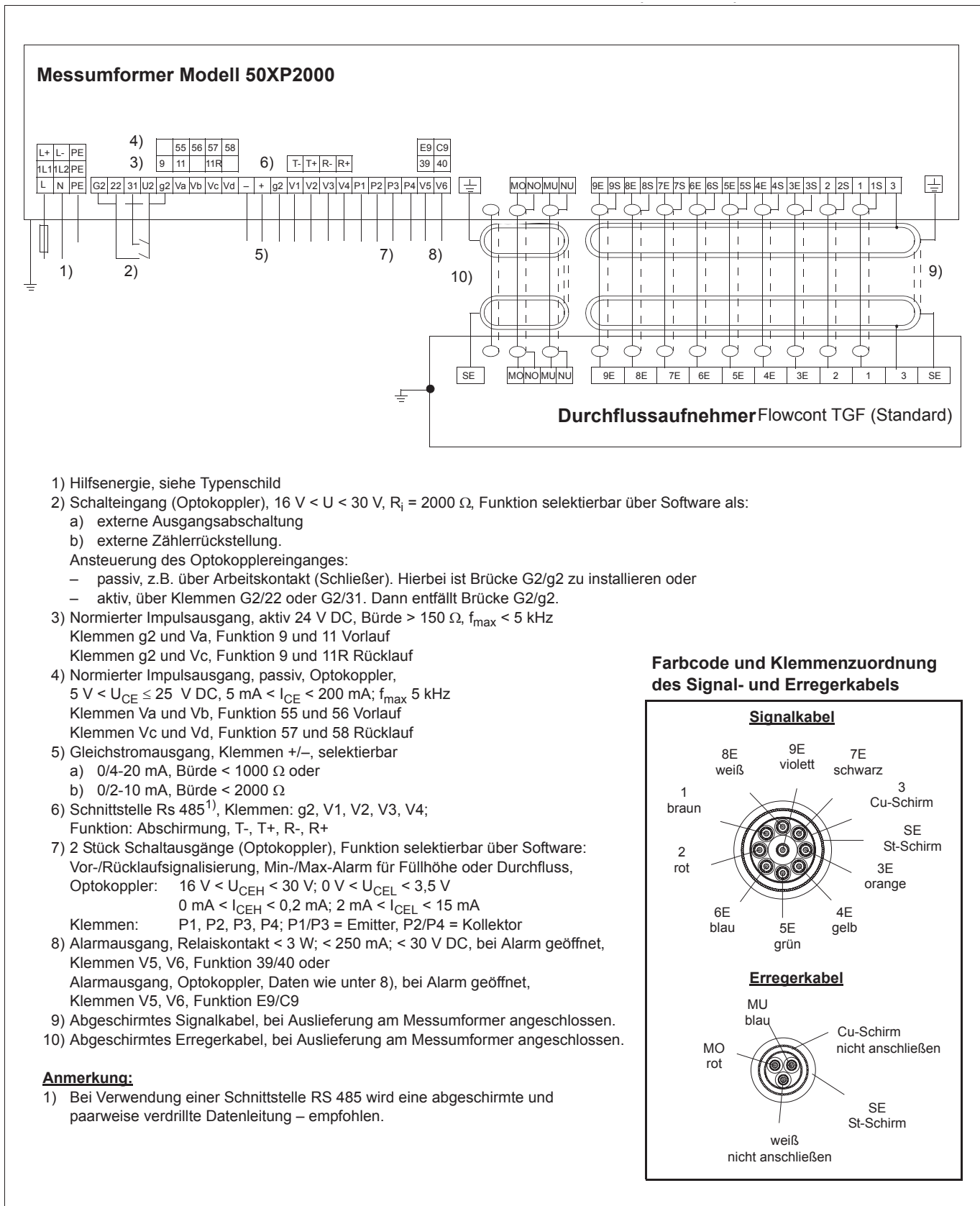
Abb. 44 Anschlussplan, Messumformer 50XP2000, Aufnahme Flowcont TGF (Standard)
