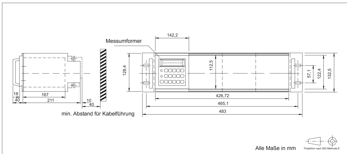
Abb. 26 Maßzeichnung, 19"-Technik
