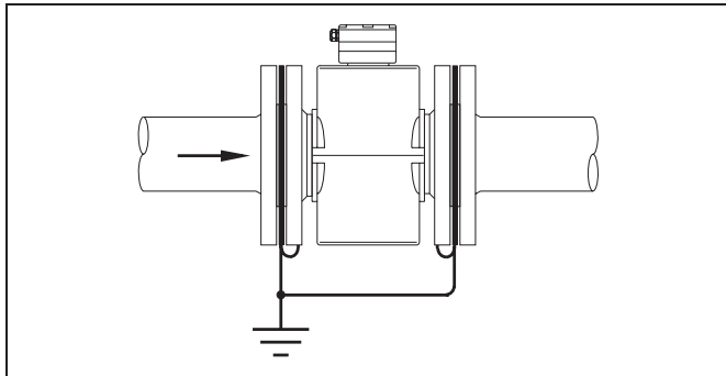
Abb. 30 Aufnehmer DN 150 bis 250, Zweischalengehäuse mit Festflansch
