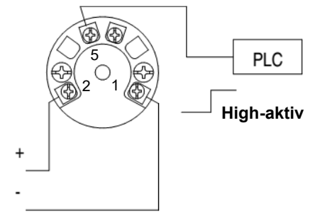
Digitaler Ausgang
