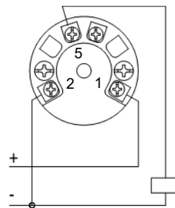
PNP Ausgang
