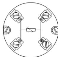
Einzelelement, 4-Leiter
