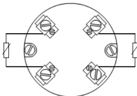
Elément double
