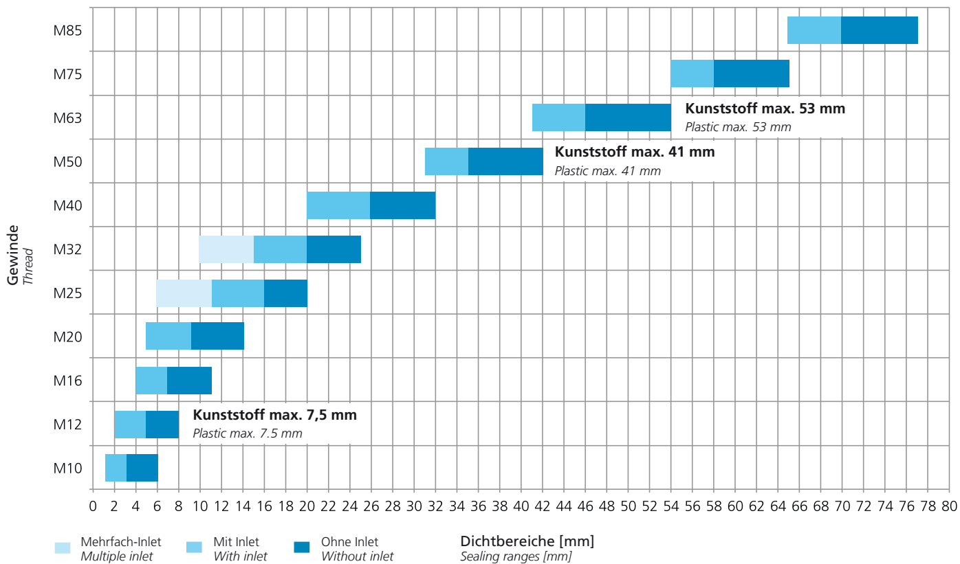
Dichtbereiche der blueglobe Sealing ranges of blueglobe
