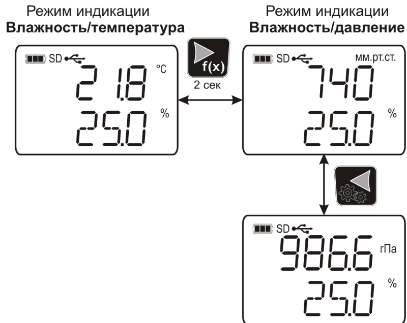
Рисунок 5.2 Переключение режимов индикации ИВТМ-7 К-Д-1
