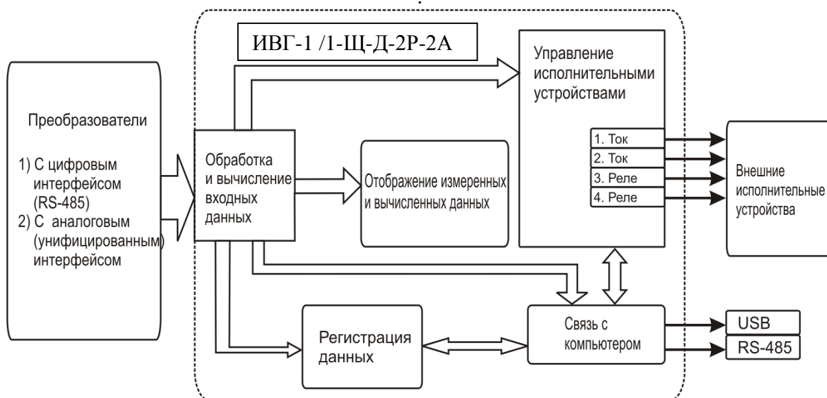
Рисунок 3.8 Структурная схема работы прибора
