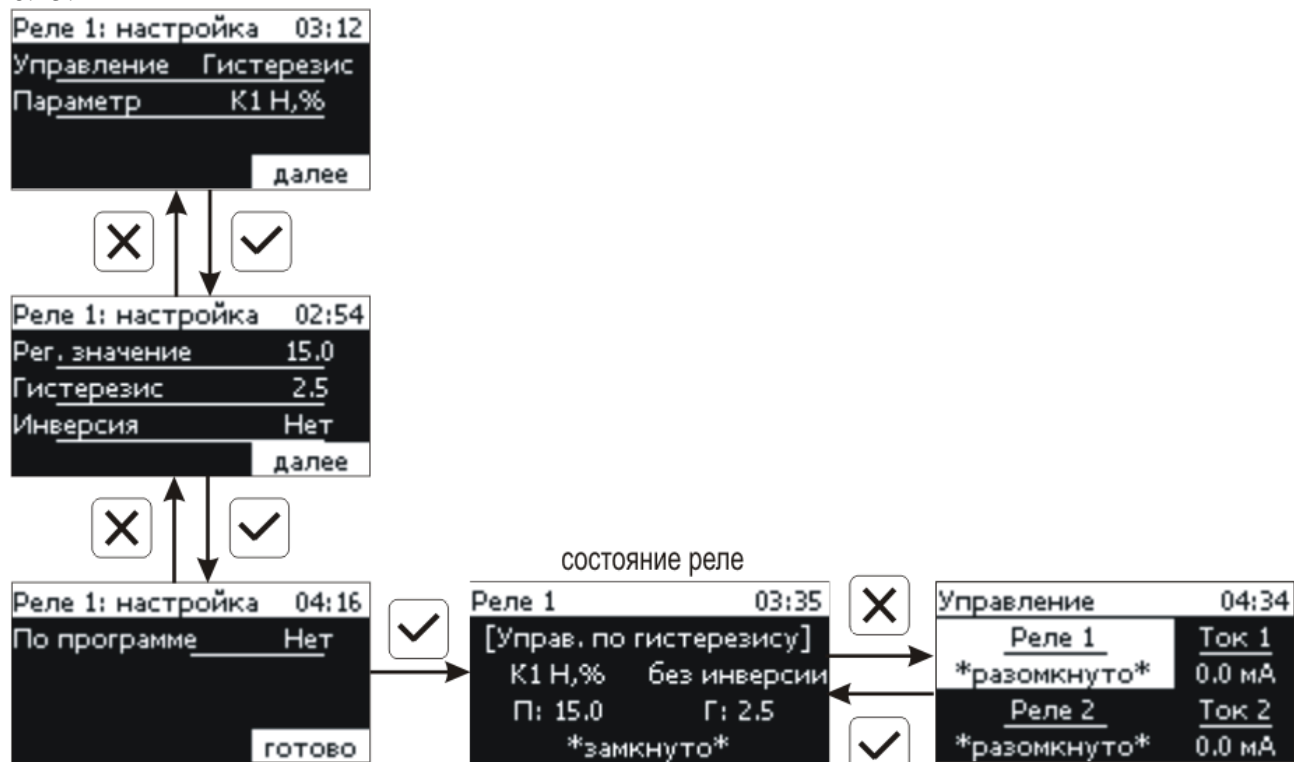
Рисунок 6.15 Настройка управления по гистерезису.
