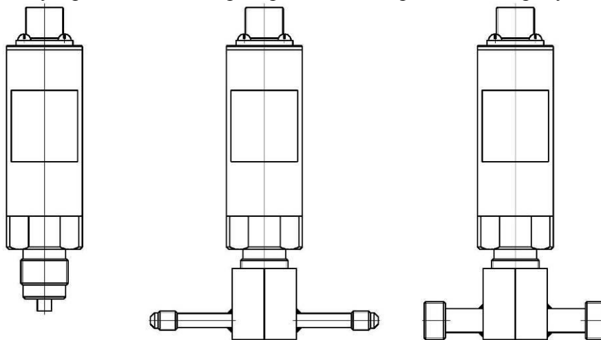
Рисунок 3.14 Измерительные преобразователи давления ИПД-02, ИПД-02-М8, ИПД-02-М16 (по порядку слева направо)
