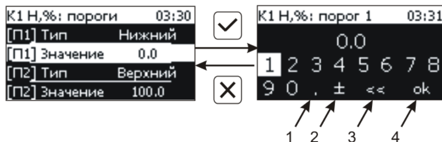
Рисунок 6.6 Экран ввода значения порога
