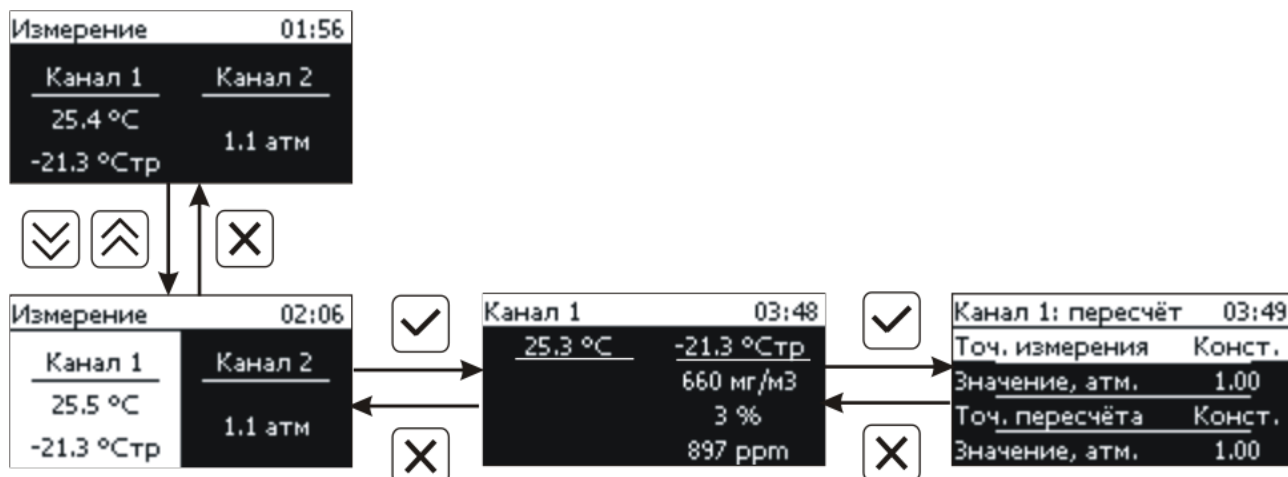
Рисунок 6.9 переход к экрану настроек пересчета влажности.
