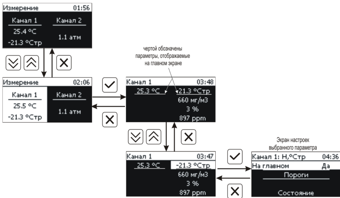
Рисунок 6.2. Структура меню канала измерения.
