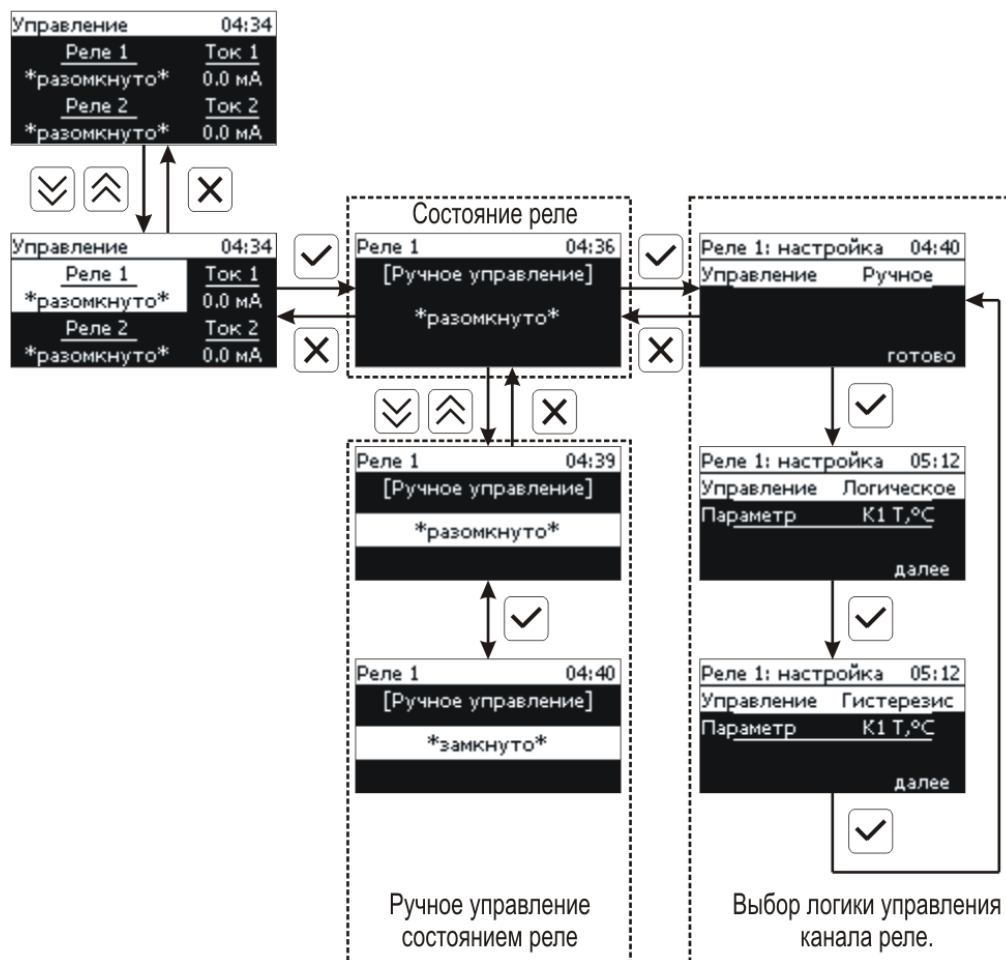
Рисунок 6.12 Выбор логики канала реле.
