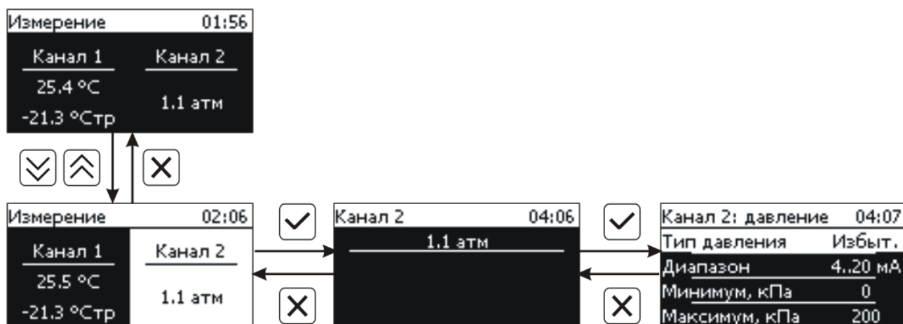
Рисунок 6.7 Вид экрана настройки параметров датчика давления
