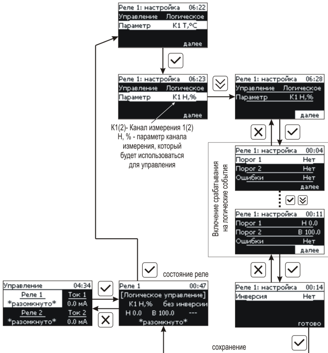
Рисунок 6.13 Настройка логического сигнализатора канала реле.
