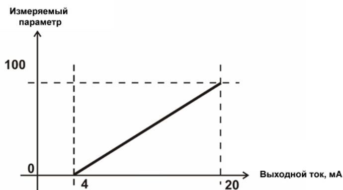
Рисунок 3.12 Линейный выход 4...20 мА по параметру от 0 до 100
